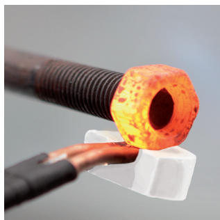
Sbloccaggio bulloni
